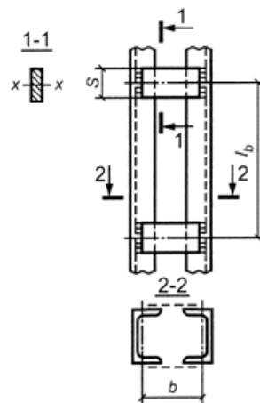
Рисунок 3 - Схемы решеток сквозных стержней
