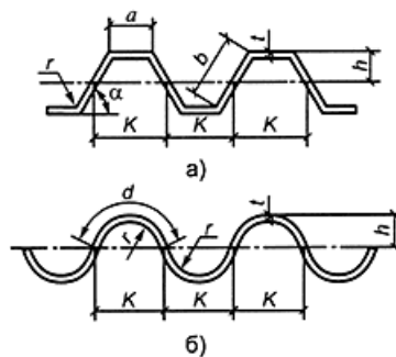
Рисунок 13 - Расчетная схема сжатого гофрированного листа
